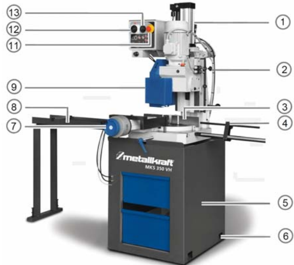
Abb. 4: Gerätebeschreibung MKS 350 VH
